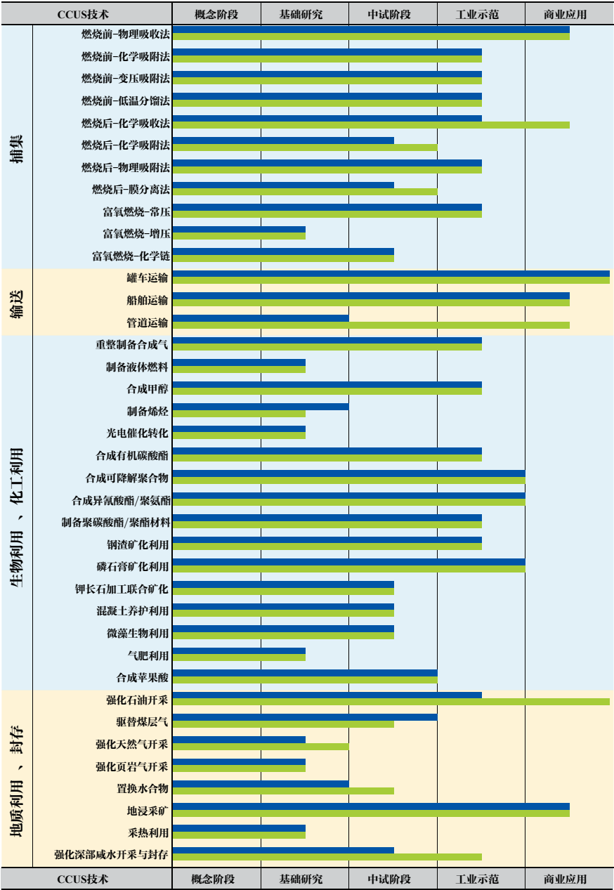
图例 国内 国外 图 8 中国 CCUS 技术类型及发展阶段
